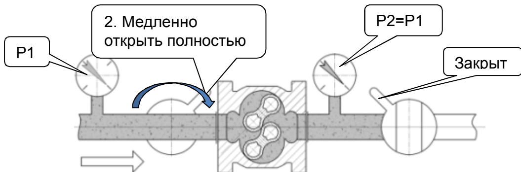
Рисунок 6 – Полное открытие запорного устройства до счетчика
