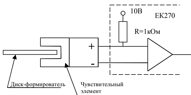
Рисунок 14 – Схема среднечастотного датчика импульсов R300
