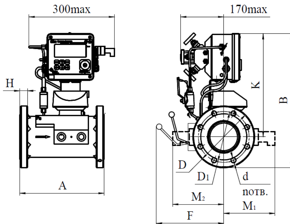
Рисунок 4.1 Направление потока газа: слева – направо (Ду200...Ду300)
